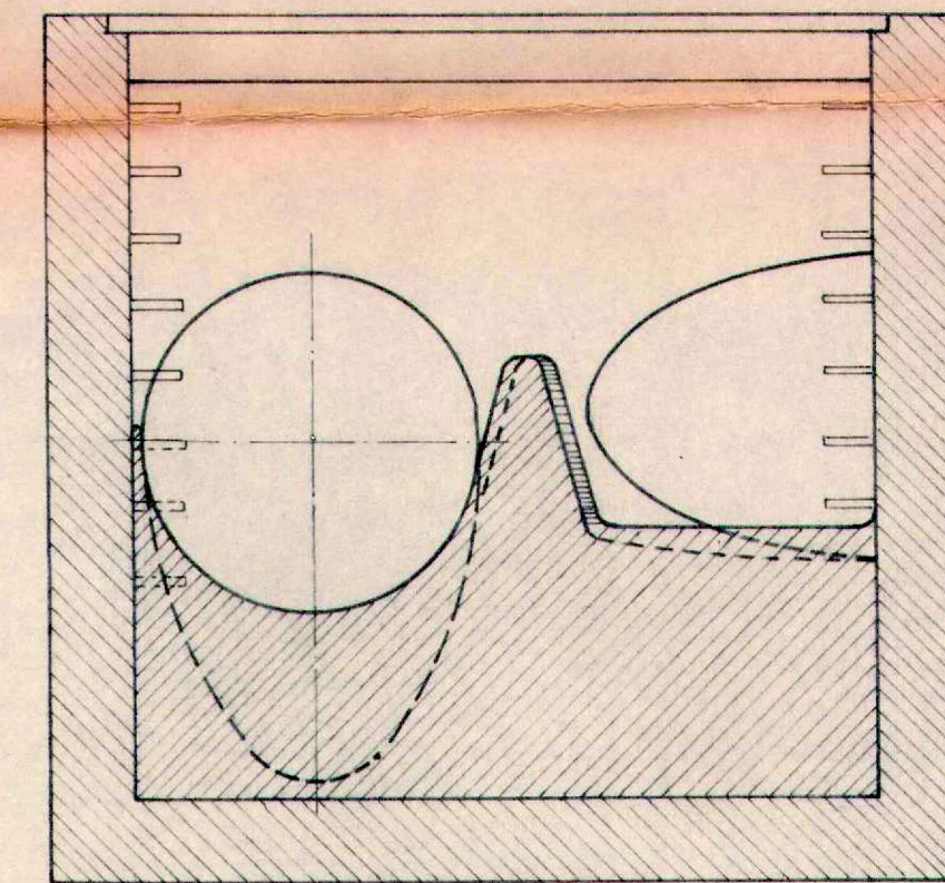
SCHNITT B - B
